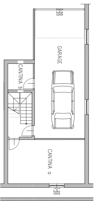
PLANIMETRIA GENERALE
